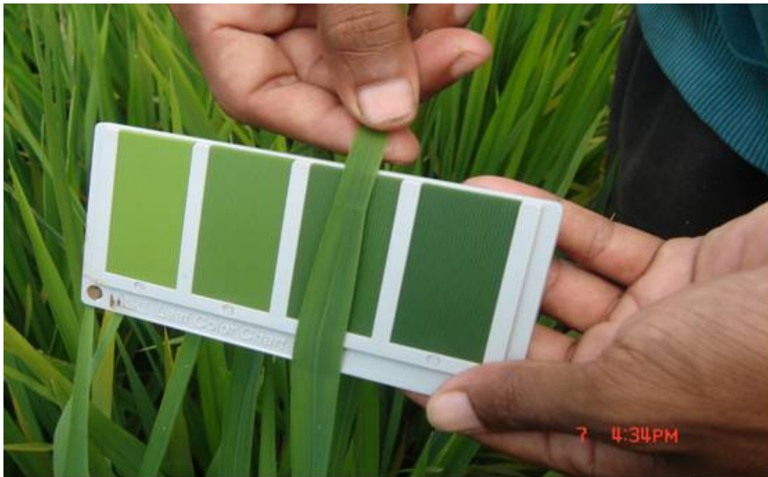
Gambar 1. Penggunaan Bagan Warna Daun, untuk mengukur warna daun dalam penetapan pemupukan N pada tanaman padi..
